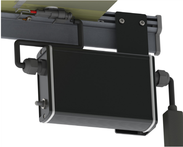
Bild oben: 2-polige Steckverbindung als Zuleitung in das Tuch
